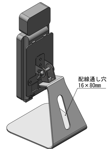
仕様図: カウンタースタンドIRC-TCSV1
