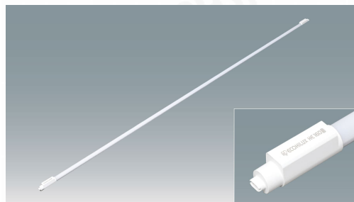
直管LEDランプ ECOHiLUX HE160S (片側給電) リニューアル
