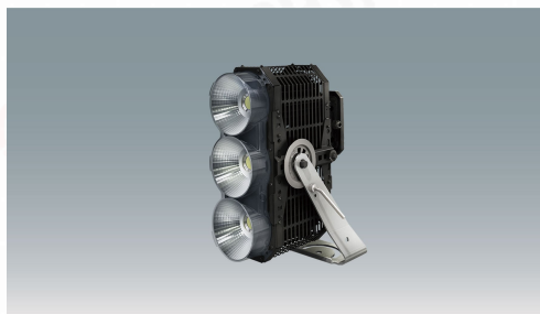
LED投光器 大光量タイプ HW-F
