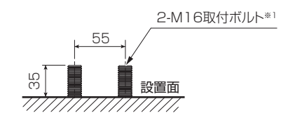
LEDモジュール2~8灯の取り付け例
