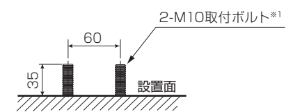
LEDモジュール1灯の取り付け例
