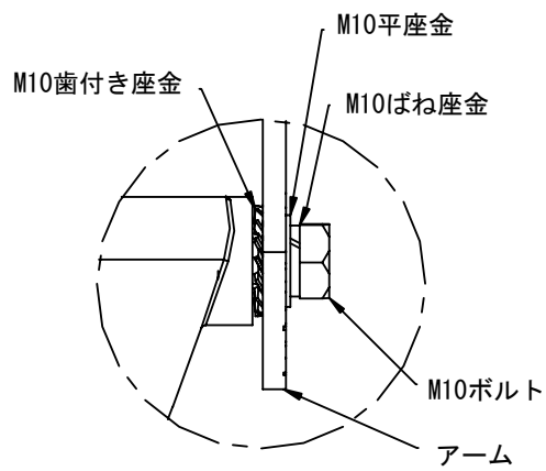
本体取付部詳細
