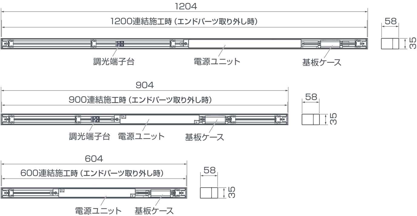
取付寸法図（背面図：取り付け面側）
