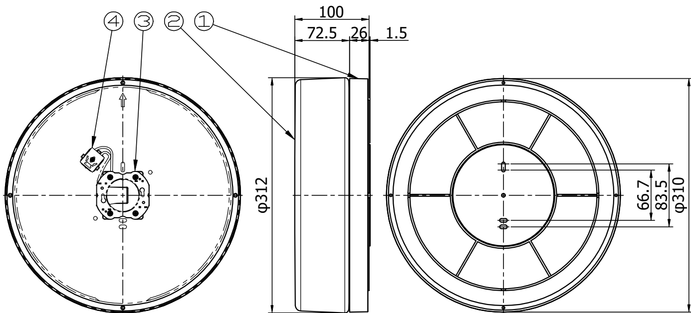
取付寸法図
