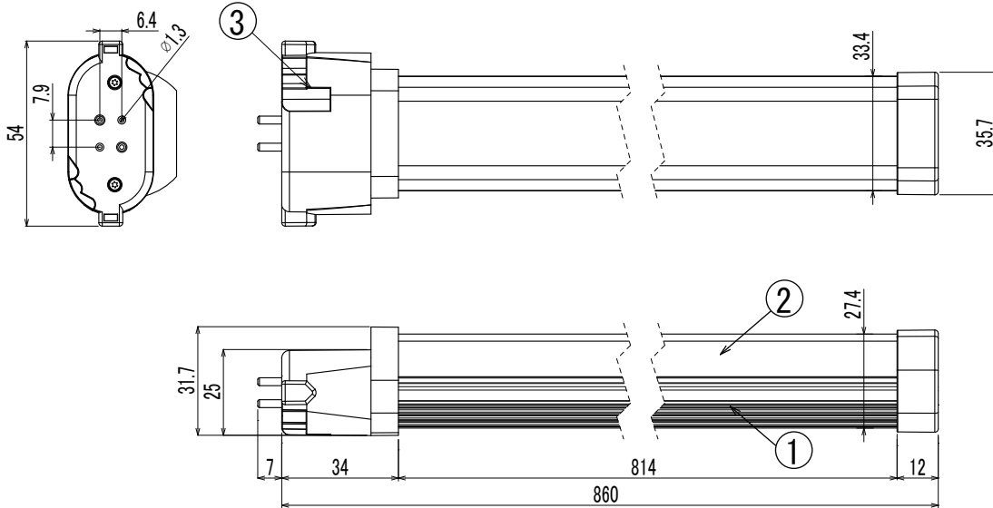
【種別】コンパクト蛍光灯代替LEDランプ96形 電源内蔵
