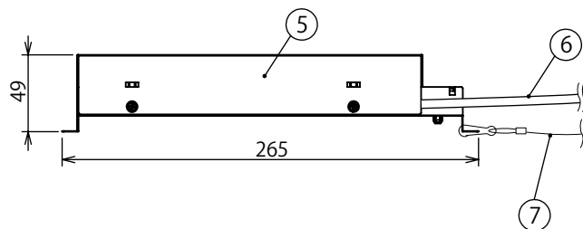
調光端子台
