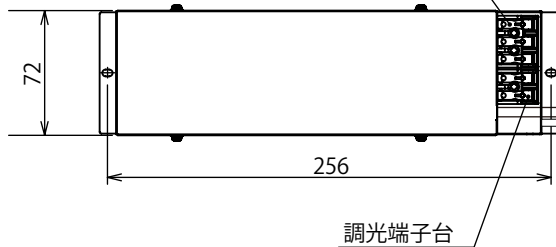
調光端子台
