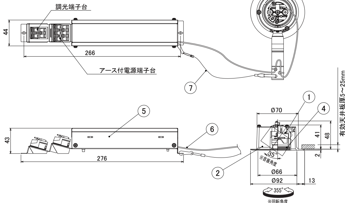
【埋込穴寸法】
