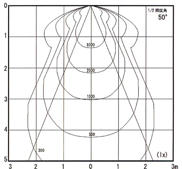
水平特性
