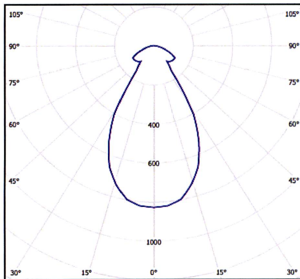
配光特性
