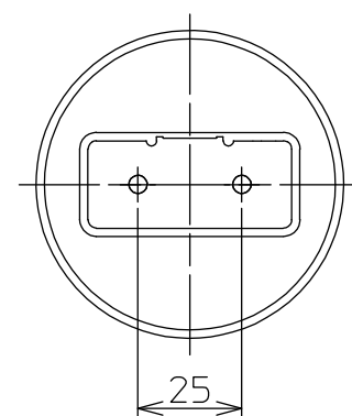
取付部詳細
