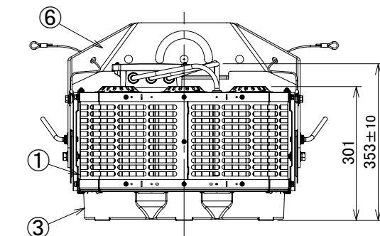
取付部詳細
