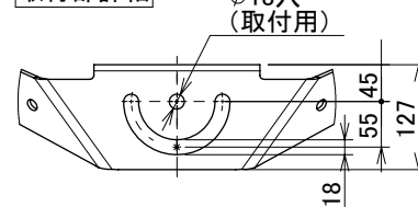
取付部詳細
