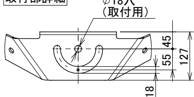
取付部詳細
