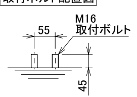
取付ボルト配置図
