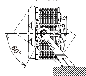
水平取付
