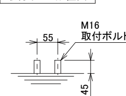
取付ボルト配置図
