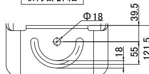
取付部詳細
