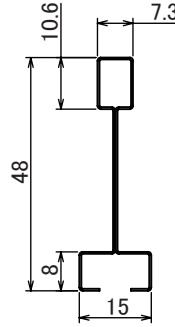
適合Tバー詳細 パナソニック:15D
