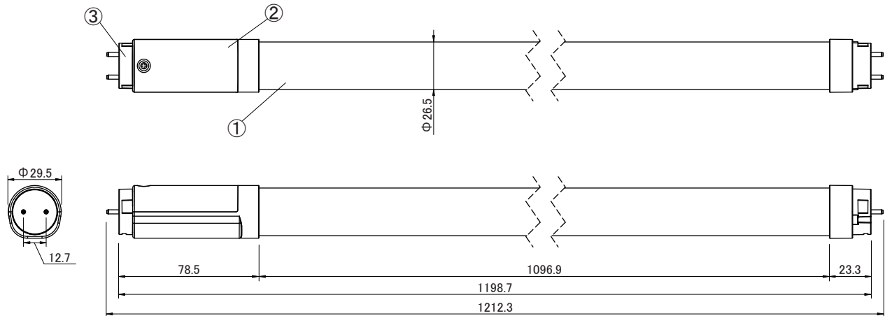
【種別】直管LEDランプ 32形
