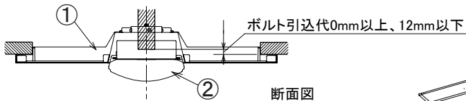
断面図
