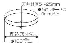
【埋込寸法】
