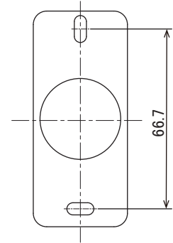
取付寸法図
