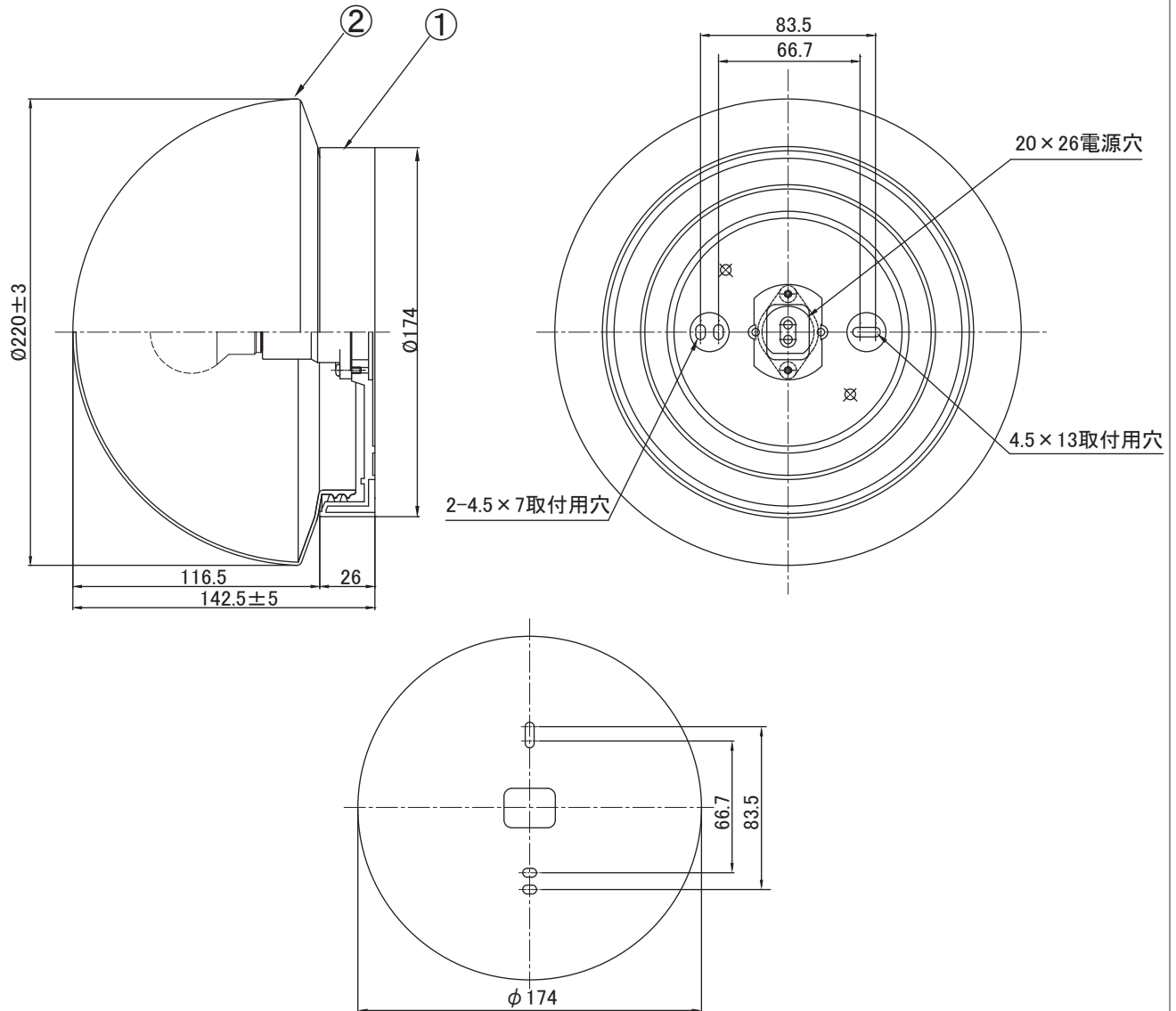
取付寸法図
