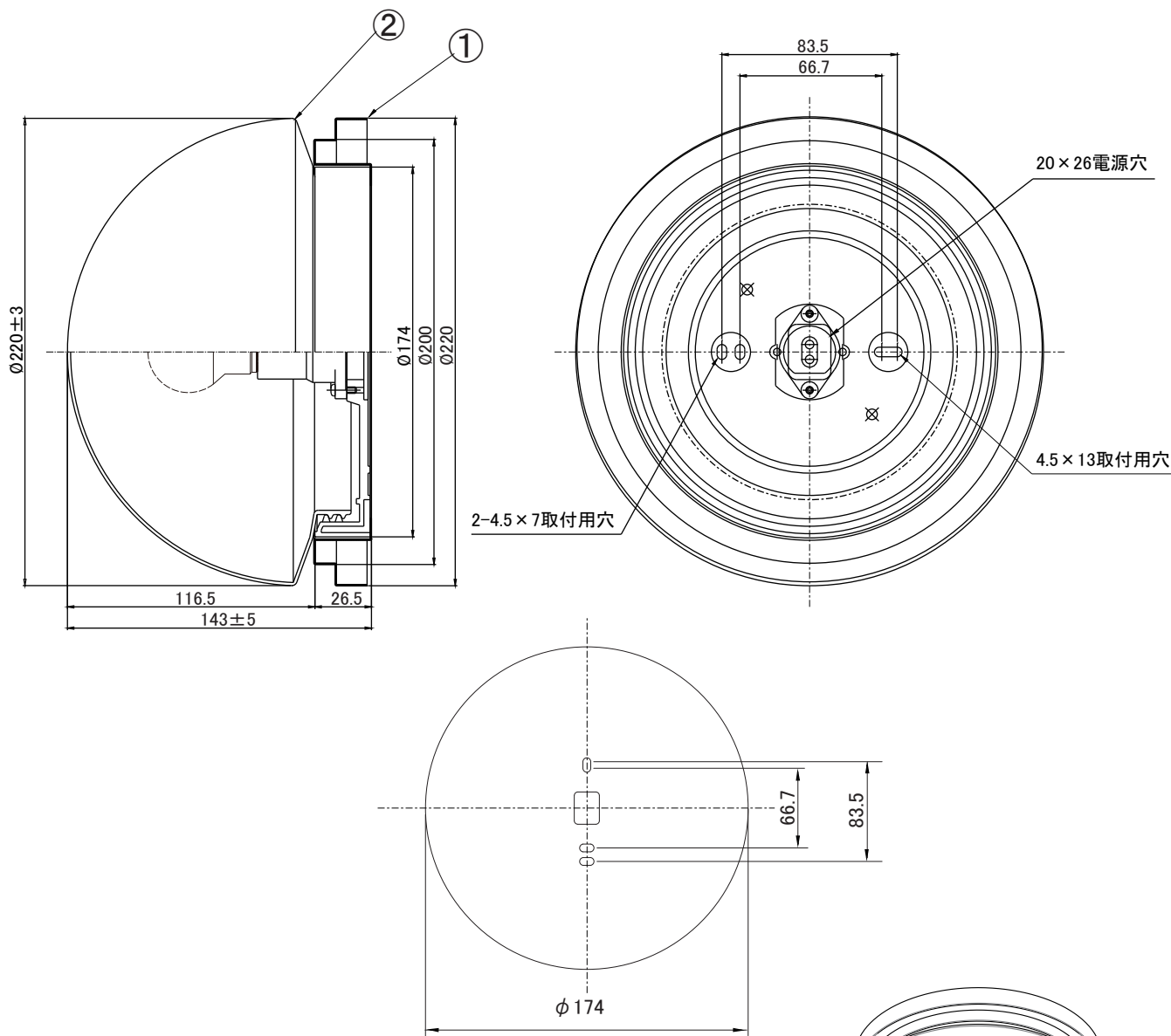
取付寸法図
