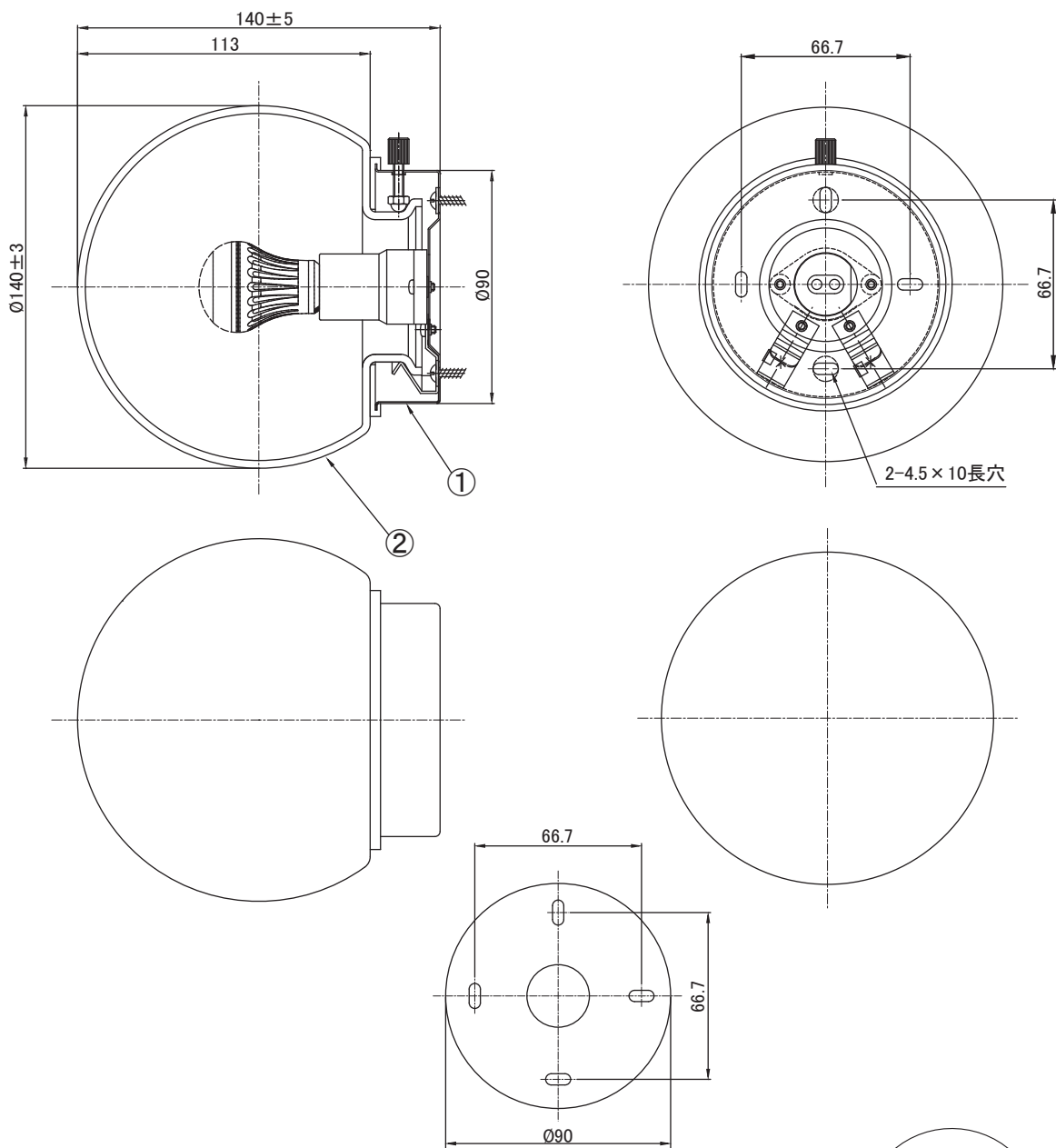
取付寸法図
