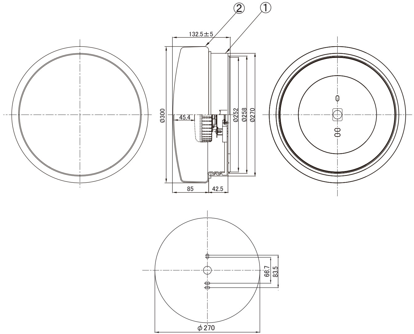
取付寸法図
