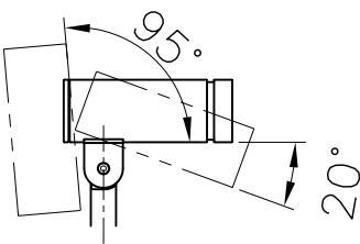
可動範囲
