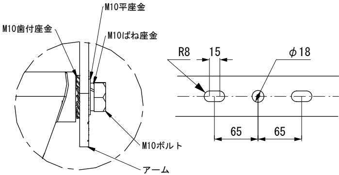
A:本体取付詳細
