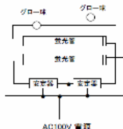
グロー式 2灯
