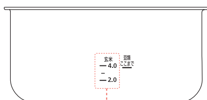
玄米の水位目盛
