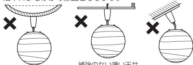
簡単にたわむ天井 補強のない薄い天井 傾斜天井
