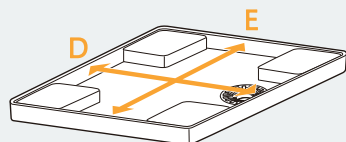
台付き防水パン
